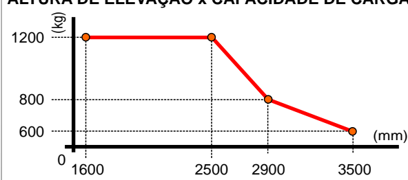
ALTURA DE ELEVAÇÃO x CAPACIDADE DE CARGA
